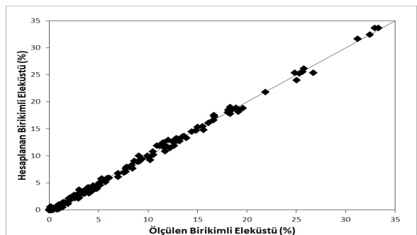
Şekil 10. Ölçülen hesaplanan birikimli elek üstü değerleri (Test 1)
