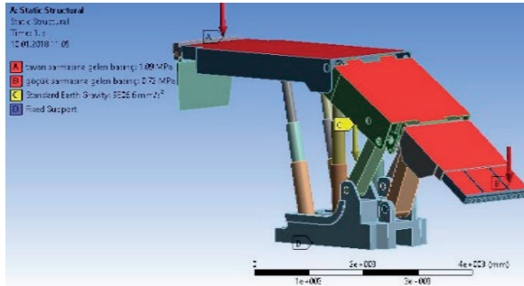
Şekil 5. Basıncın ana göçük sarmasına uygulanması
