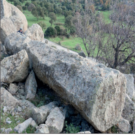
Şekil-5 V Tipi ve Üçlü Kama Kesim İzleri
