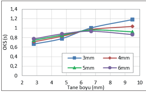
Şekil 7. Tanelerin farklı titreşim genliklerindeki ortalama kalma süreleri
