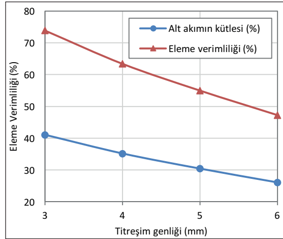
Şekil 5. Titreşim genliğinin eleme verimliliği ve alt akımın kütlelerine etkileri
