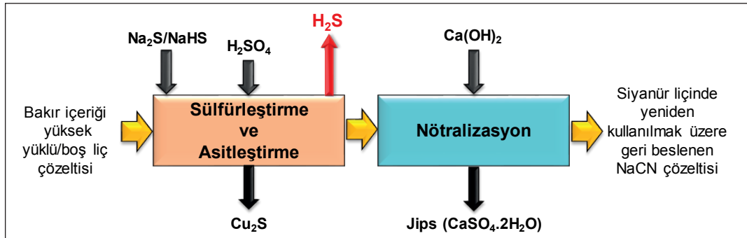
Şekil 5. SART prosesi şematik akım şeması (Nodwell vd. (2012)'den değiştirilerek)
