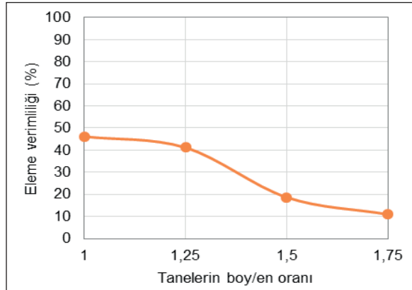
Şekil 24. Farklı boy/en oranlarına sahip olan tanelerle yapılan simülasyonların eleme verimlilikleri
