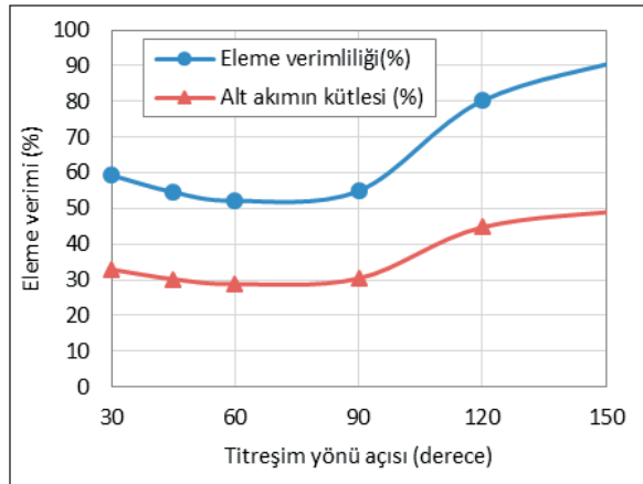
Şekil 12. Titreşim yönünün eleme verimliliği ve alt akımın kütledeki etkileri
