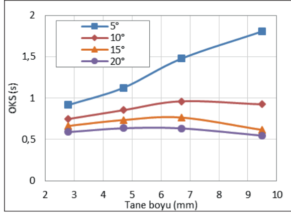
Şekil 4. Tanelerin farklı elek eğimlerinde ortalama kalma süreleri
