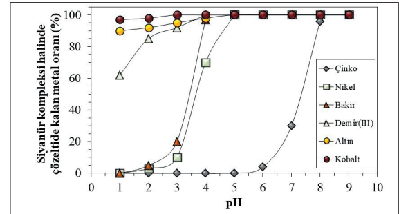
Şekil 3. Metal-siyanür komplekslerinin kararlılığının pH'ya göre değişimi (Her bir metalin toplam derişimi = 10^{-4} M, 20^\circ\text{C} ) (Fleming ve Cromberge, 1984)
