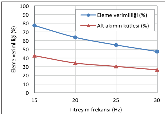
Şekil 8. Titreşim frekansının eleme verimliliği ve alt akımın kütesine etkileri
