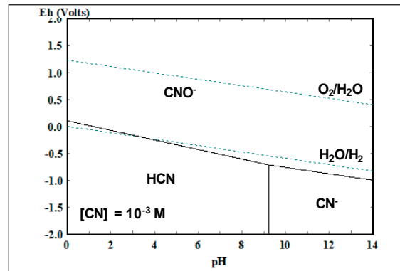
Şekil 1. \text{CN-H}_2\text{O} sistemine ait Eh-pH diyagramı ( [\text{CN}^-] = 0,02 \text{ M} ) (HSC Chemistry, 2011).
