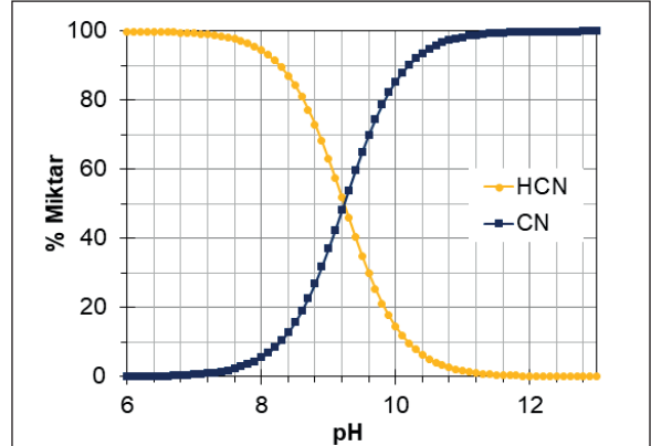
Şekil 2. HCN ve \text{CN}^- oluşumunun çözeltinin pH değerine göre değişimi (Logsdon vd., 2001)
