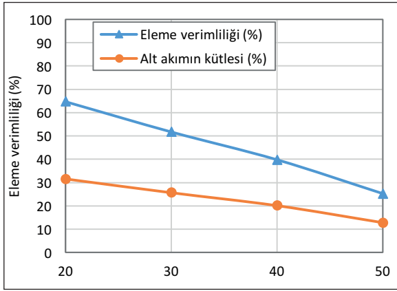
Şekil 20. Farklı yakın boyutlu malzeme içeren beslemelerin eleme verimlilikleri ve alt akım kütleleri
