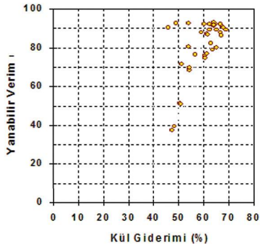
Şekil 8. Aglomerasyonda çeşitli parametrelerin yanabilir verim ve kül giderimi üzerine etkisi.
