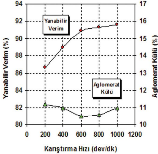
Şekil 6. Aglomerasyonda karıştırma hızının yanabilir verim ve aglomerat külüne etkisi (%15 yağ ilavesi).
