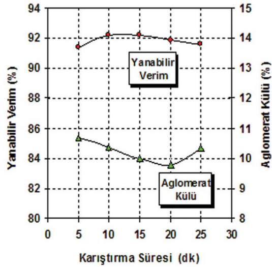
Şekil 7. Aglomerasyonda karıştırma süresinin yanabilir verim ve aglomerat külüne etkisi (%15 yağ ilavesi).
