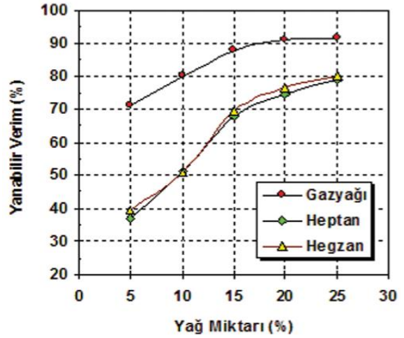
Şekil 3. Aglomerasyonda farklı bağlayıcı yağların yanabilir verime etkisi.
