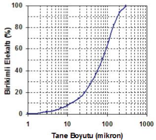
Şekil 2. Aglomerasyon deneylerinde kullanılan örneğin tane boyut dağılımı.
