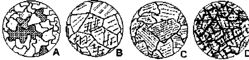
Şekil 1. Mermerlerde tane boyutu ve tane sınırları ilişkileri: (A) ince taneli ve tane sınırları dantel gibi girintili çıkıntılı, (B) iri taneli ve tane sınırları düzgün, (C) iri taneli ve tane sınırları dantel gibi girintili çıkıntılı, (D) ince taneli ve tane sınırları düzgün (Sarıışık, Çelik, ve Gürcan, 2003).
