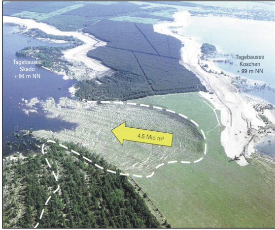
Şekil 1. Koschen-Skado linyit açık işletmeleri şev duraysızlığı örneği (LMBV, 1996)
