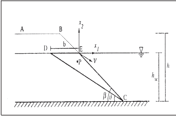
Şekil 4. Şev geometrisi ve parametrik büyüklükler (Raju,1994)
