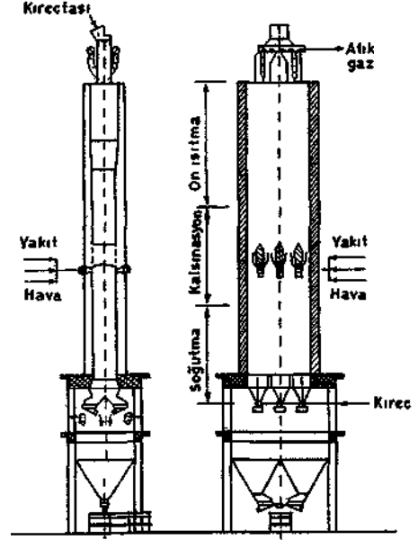
Şekil 2 Bir dik fırının şematik gösterimi
