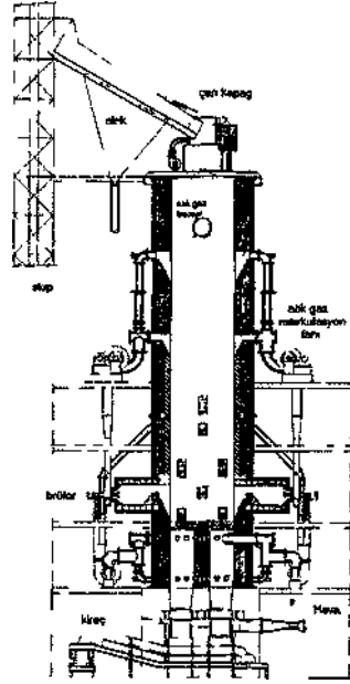
Şekil 1 AZBE yüksek kapasiteli dik fırın (150-250 t/gun) (BOYNTON R S , 1980)
