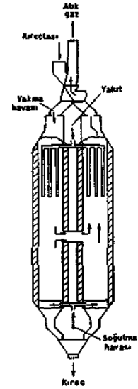
Şekil 4 Maerz fırını şematik gösterimi
