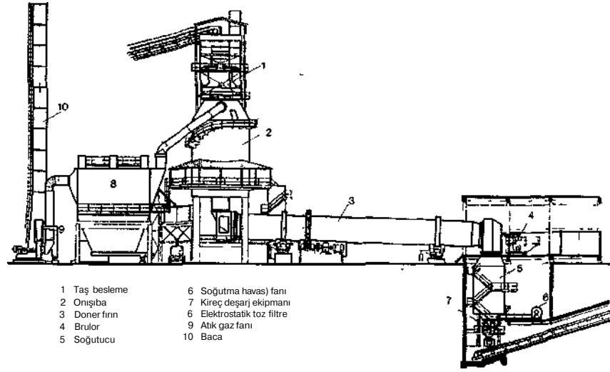
Şekil 5. Önıştmah döner kireç fırını (WİEMERKJH., 1975)
