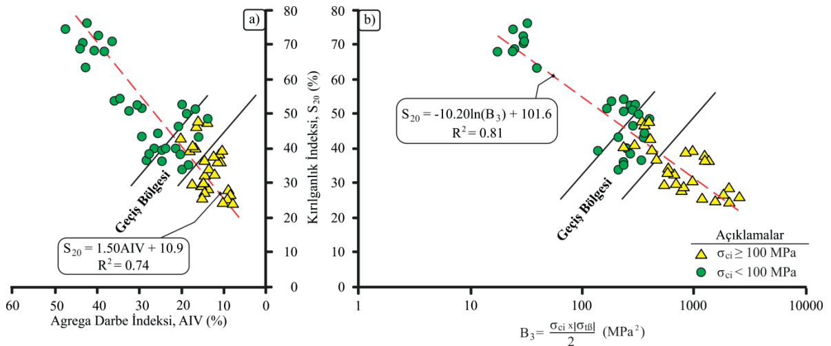
Şekil 5. a) AIV ile S_{20} arasındaki ilişki b) B_3 kırılmalık indeksi ile S_{20} arasındaki ilişki.
