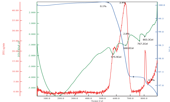
Şekil 2. Talkın DTA/TG analiz sonuçları
