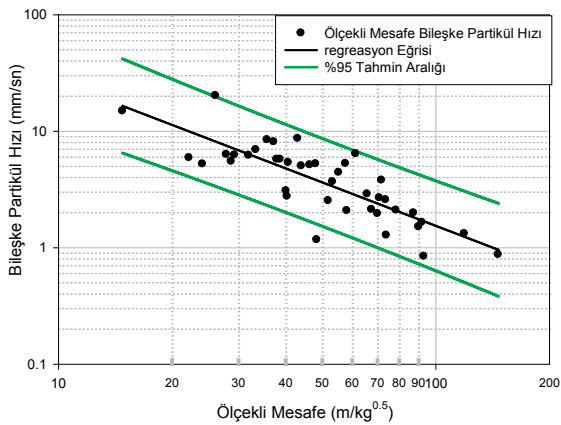
Şekil 4 İncelenen bölgede ölçekli mesafe-bileşke partikül hızı ilişkisi (Karakuş vd., 2016)
