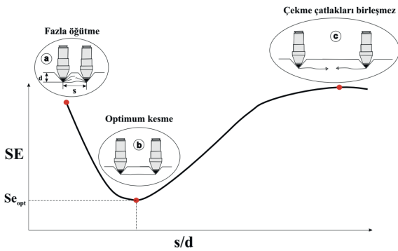
Şekil 3. s/d ile spesifik enerjinin değişimi
